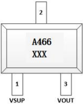
SOT23
