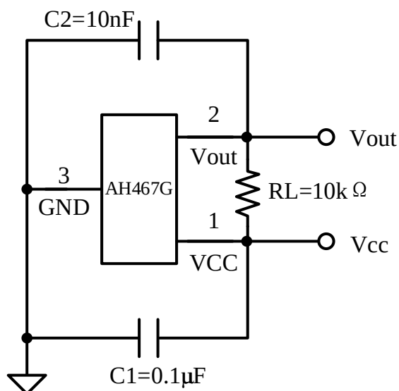
典型应用电路 1
