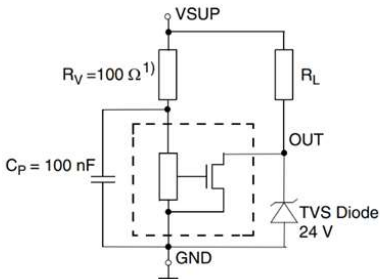
典型应用电路 3
