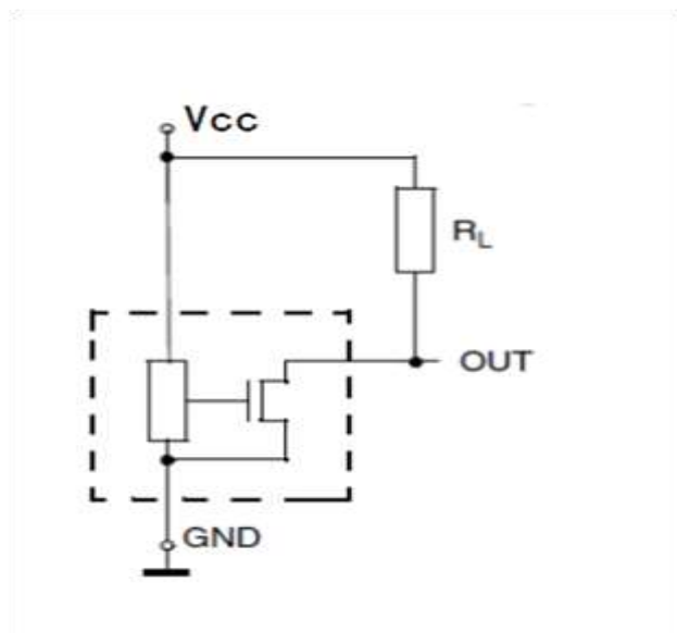
典型应用电路 1
